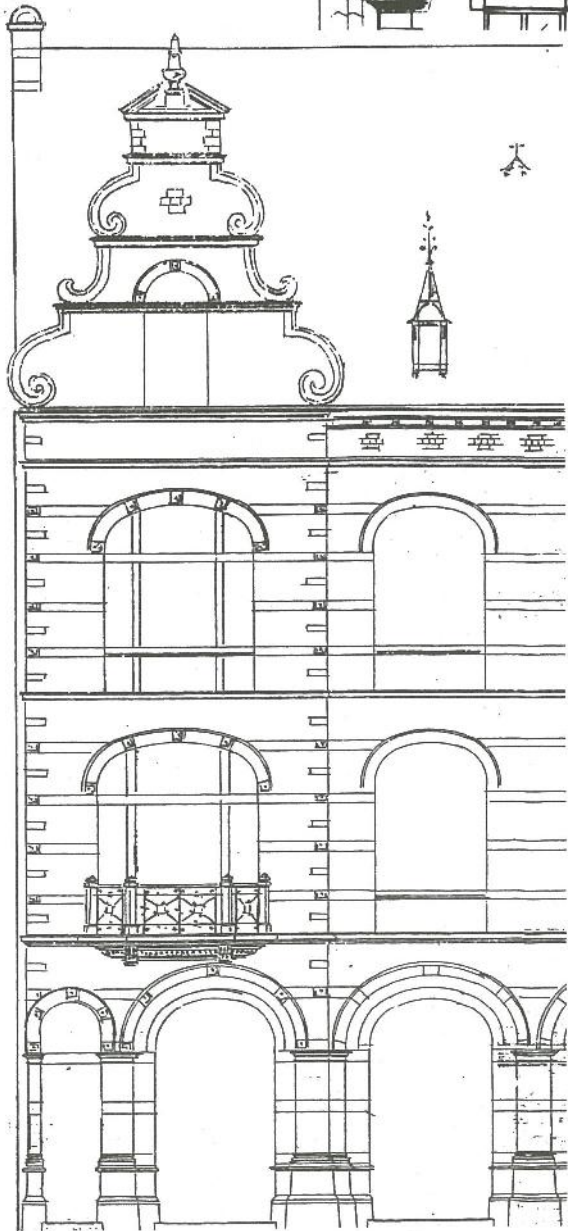
Gedeelte van het origineel plan van de voorgevel. Van deze werd afgeweken bij de uitvoering; zie topgevel (inlas)
